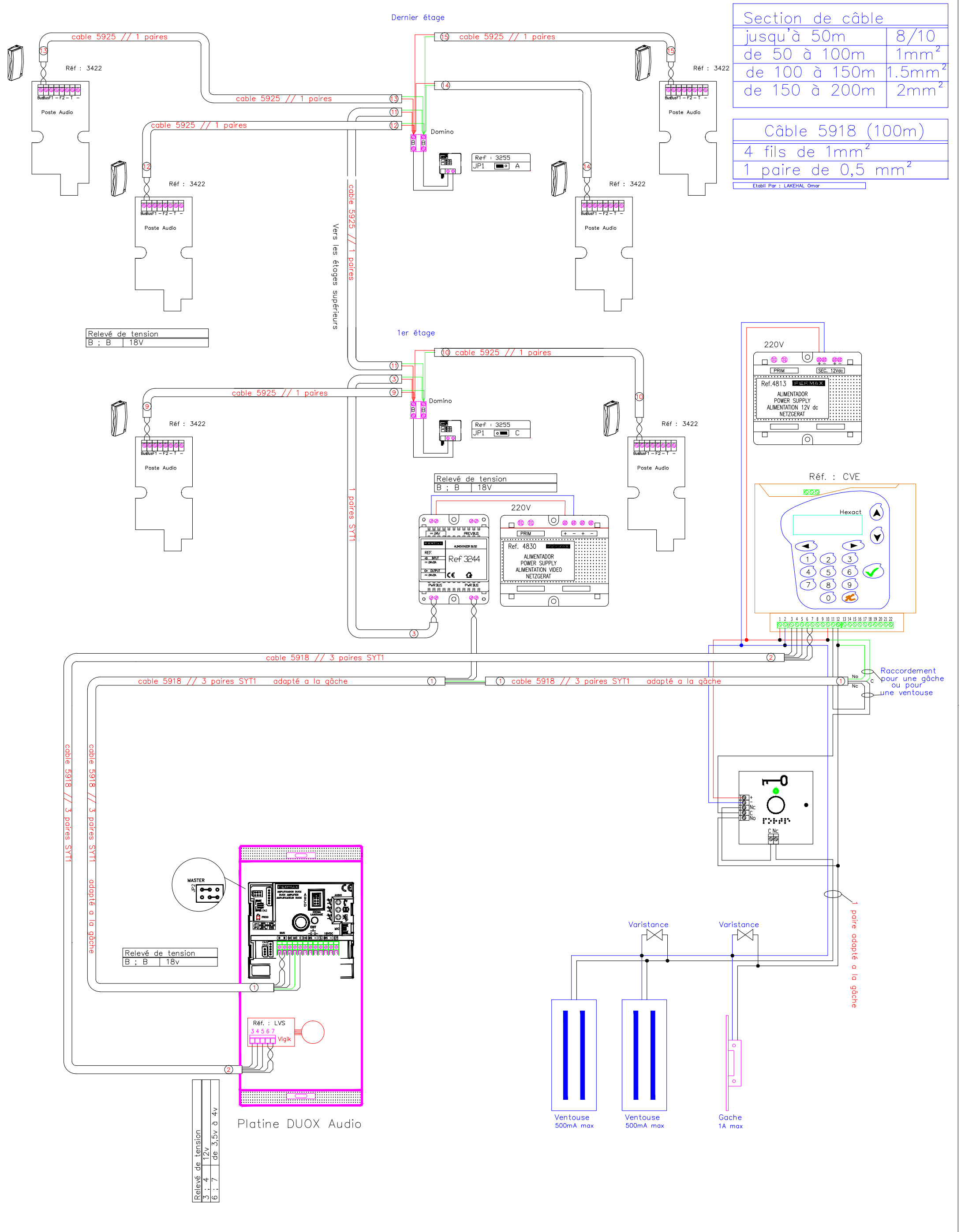
Schéma Audio DUOX avec une CVE
